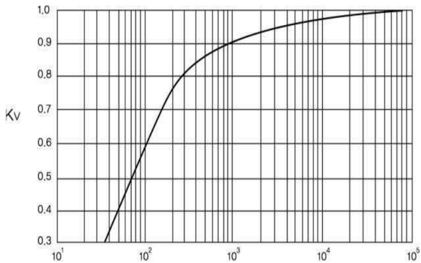
그림 2.6.1.4.2① 밸런스 벨로즈형 안전밸브 배압보정계수
