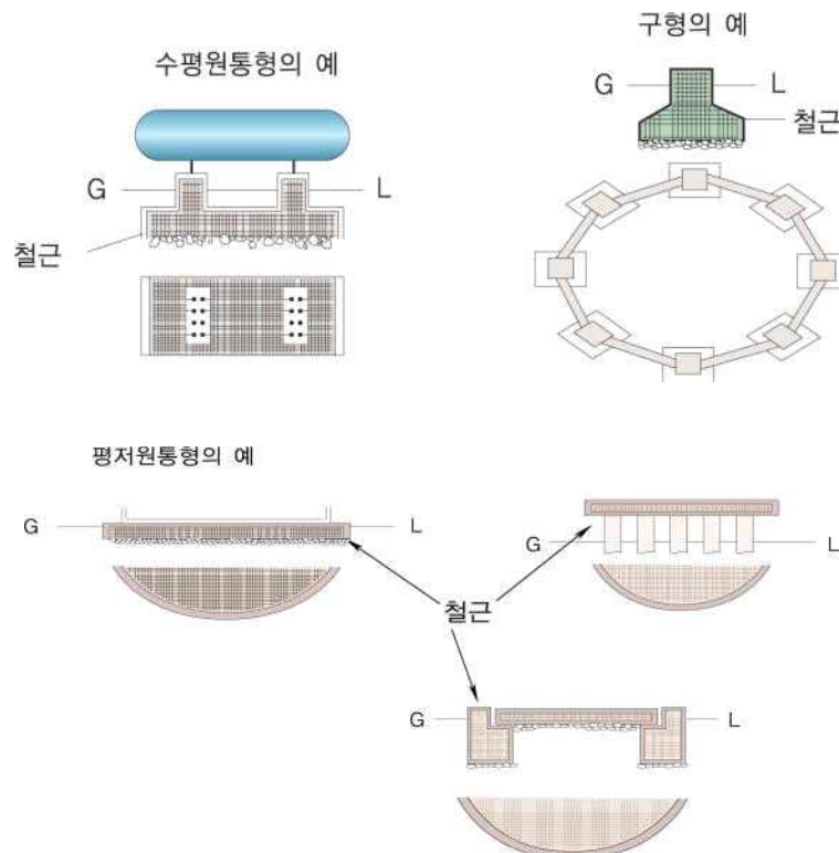
그림 2.2.2.3 저장탱크의 수평기초면
