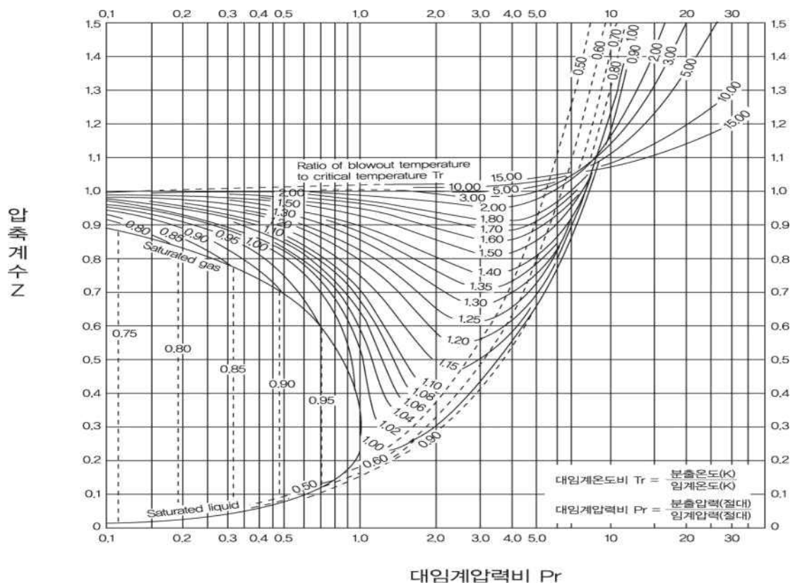
그림 2.6.1.4.1④ 압축계수
