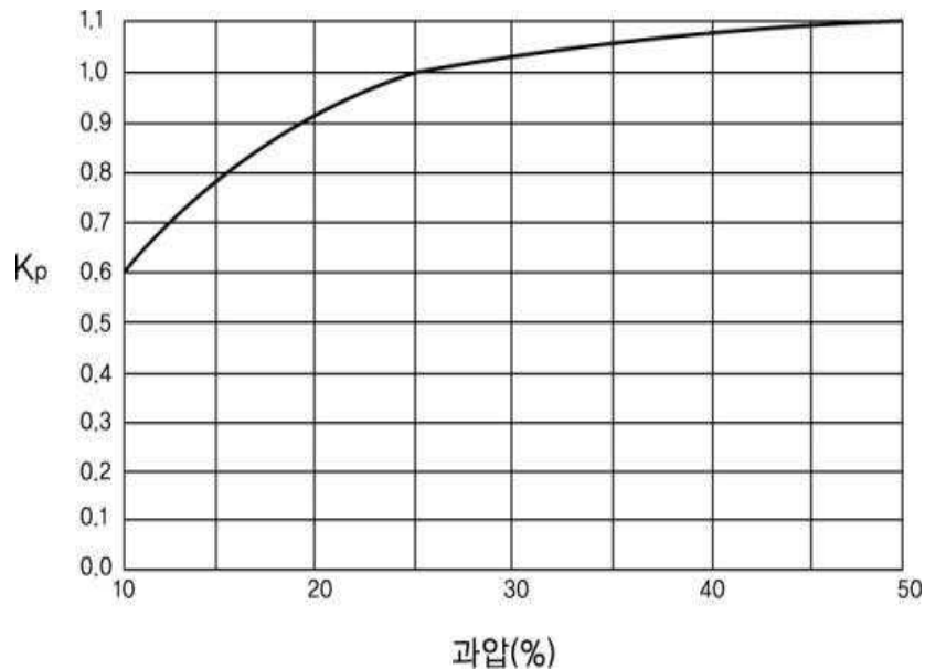
그림 2.6.1.4.2③ 과압보정계수
