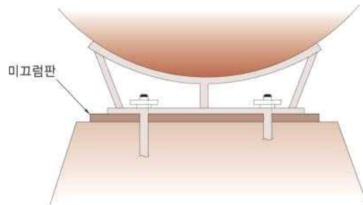
그림 2.2.3.5 미끄럼판의 설치방법
