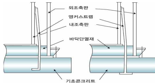
그림 2.2.3.7 평저형 수소저장설비의 앵커스트립 설치방법
