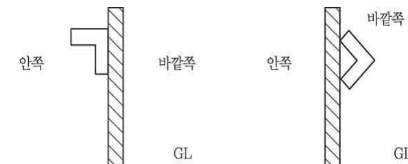
그림 2.9.2.3.2 강판제방호벽의 앵글강 보강
