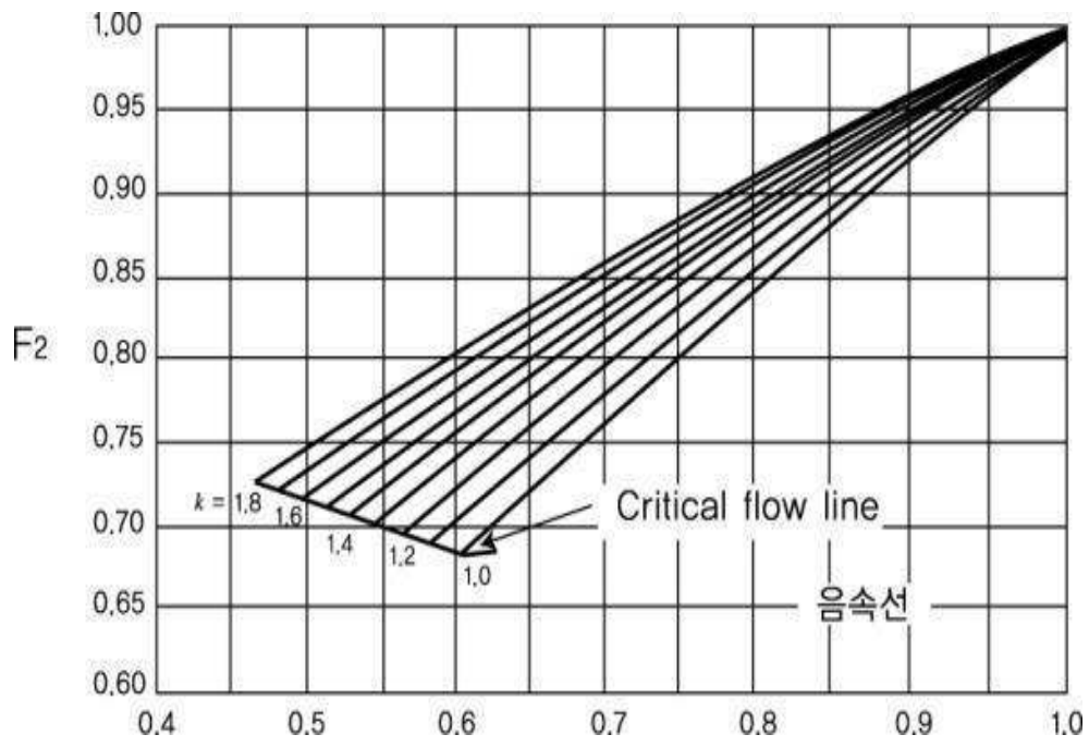
그림 2.8.1.4⑤ 이음속계수
