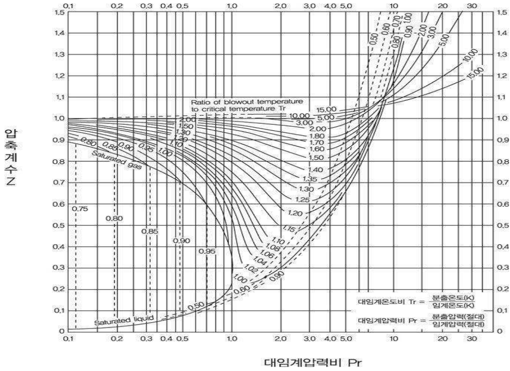
그림 2.8.1.4④ 압축계수
