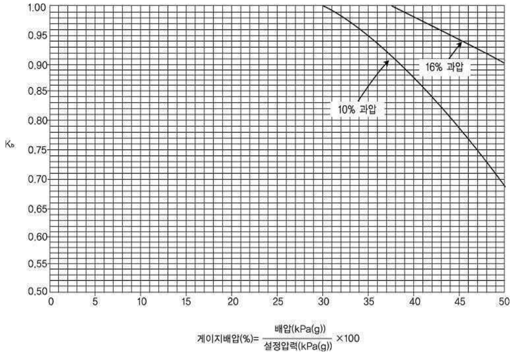
그림 2.8.1.4② 벨런스 벨로우즈형 안전밸브 배압보정계수
