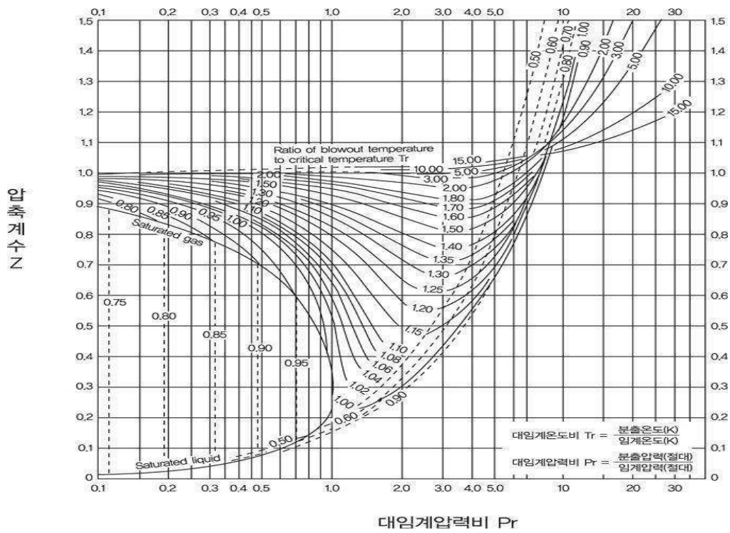
그림 2.8.1.4④ 압축계수
