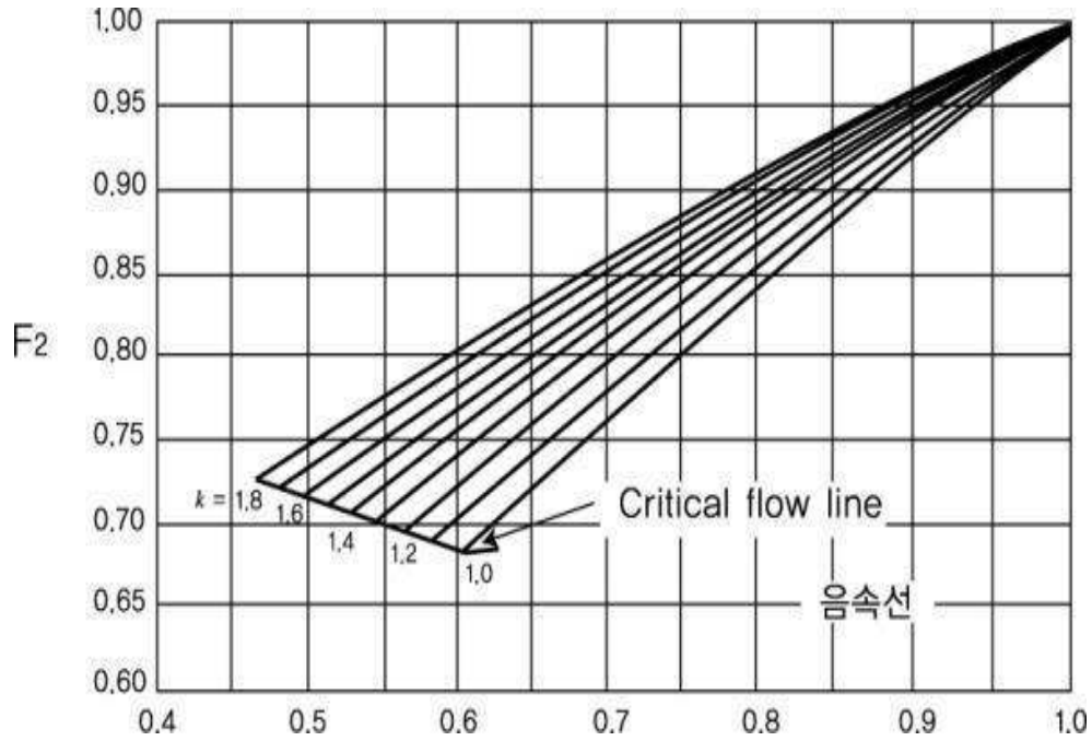
그림 2.8.1.4⑤ 이음속계수
