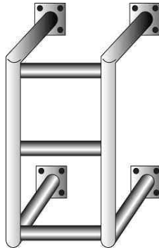
그림 2.5.7.3.1(2)② “C” 형태로 가공한 강관제 구조물에 의한 방호조치
