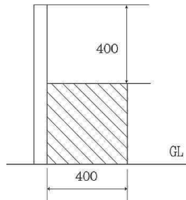
그림 2.9.2.2.3 보조벽의 높이
